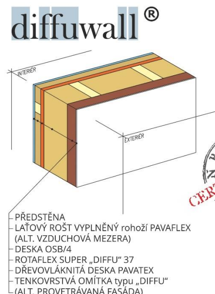
Obr. 14 : Konstrukce Diffuwall®
